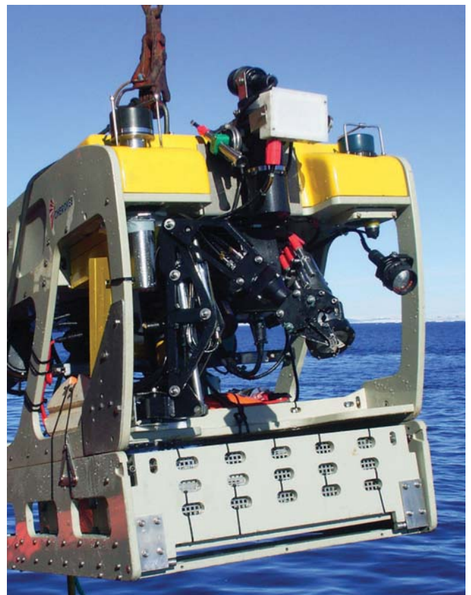
Abb. 3: Dieses ferngesteuerte Unterwasserfahrzeug liefert im Rahmen der Biodiversitätsforschung quantitative Daten gleichermaßen auf Schlamm- und Hartböden. Damit können insbesondere kleinräumige Veränderungen am Meeresboden erkannt werden (Foto: J. Gutt, AWI).
